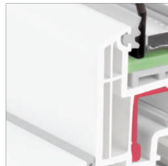
Dizajn ravnog krila
