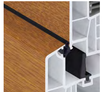
Folienkaschiertes GENE-Profil
