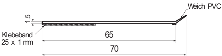
Flachleiste 70mm
